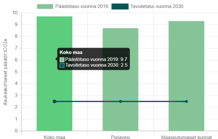
Kuva: Pielaveden päästöt laskettuna kulutusperäisellä mallilla. Tulos saatu 2024. Hiilineutraali.fi, Syke
