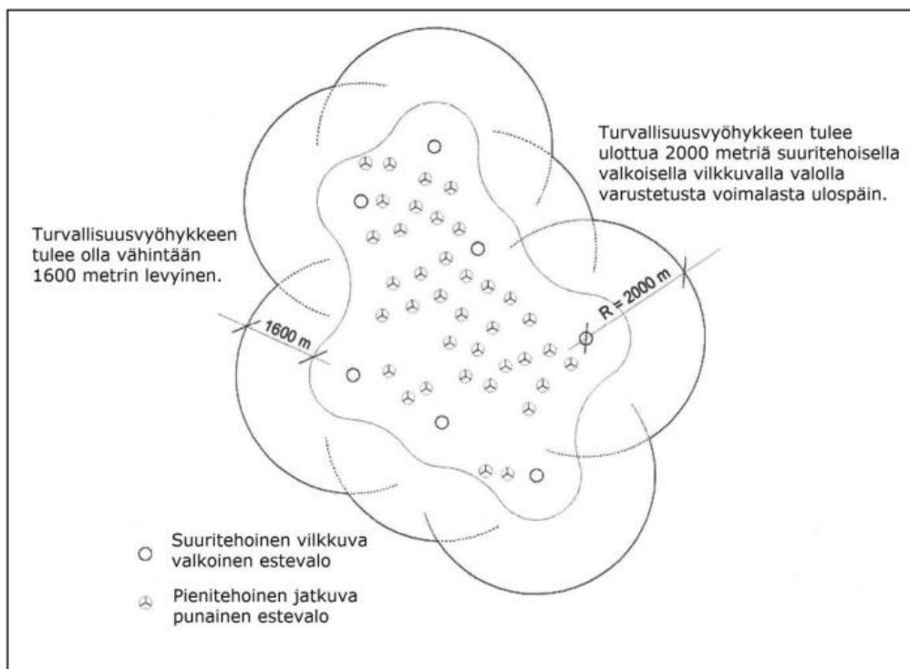
Kuva 86. Lentoestevalojen sijoitteluesimerkki, kun tuulivoimapuiston voimaloiden korkein pyyhkäisykohta on yli 150 metriä maanpinnasta. Tuulivoimaloiden ulkokehän muodostavat suuritehoiset B-typin vilkkuvat valkoiset lentoestevalot (Liikenne- ja viestintävirasto Traficom 2020).
