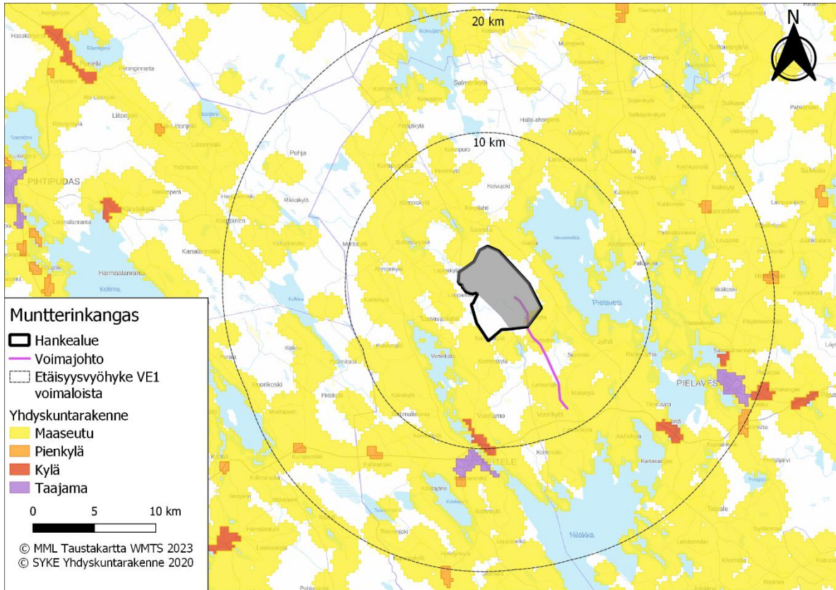
Kuva 15. Yhdyskuntarakenne kaava-alueen ja sähkönsiirtoreitin ympäristössä (Suomen ympäristökeskus 2020). Pielaveden kunnan puolelle sijoittuva osa alueesta esitetty tummennettuna.
