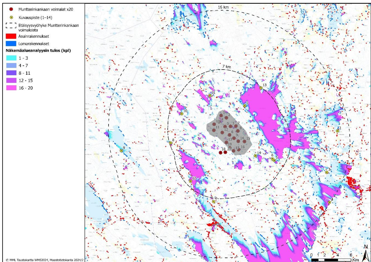
Kuva 19. Näkymäalueanalyysikartta VE1. Pielaveden kunnan puolelle sijoittuva osa alueesta esitetty tummennetulla.
