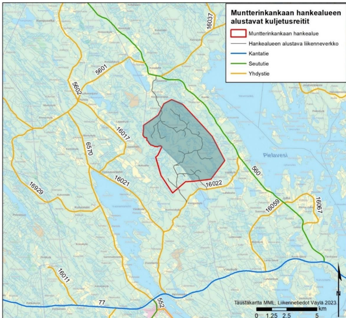
Kuva 76. Kaava-aluetta (tummennettu osa hankealueesta) ympäröivä maantieverkko ja alustavat sisäänmenoreitit.
