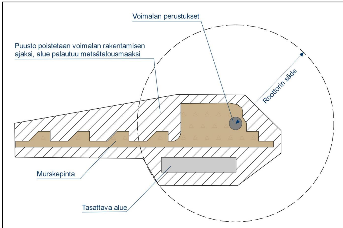
Kuva 92. Tyypillinen tuulivoimalan kokoamis- ja pystytysalue (FCG Finnish Consulting Group Oy).
