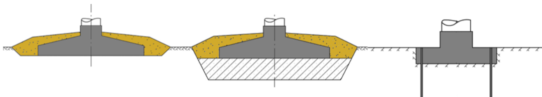
Kuva 87. Tuulivoimalat voidaan perustaa useilla eri tavoilla. Periaatekuvat maavaraaisesta teräsbetoniperustuksesta (vasemmalla), teräsbetoniperustuksesta massanvaiholla (keskellä) sekä kallioankkuroidusta teräsbetoniperustuksesta (oikealla).
